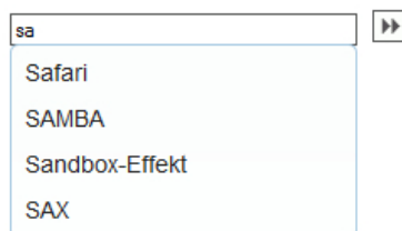
Abbildung 6-6: Autovervollständigung
